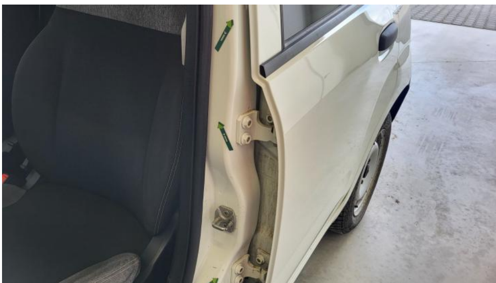
Photo 64. Słupek środkowy L - Wgniecenie/odkształcenie 1
