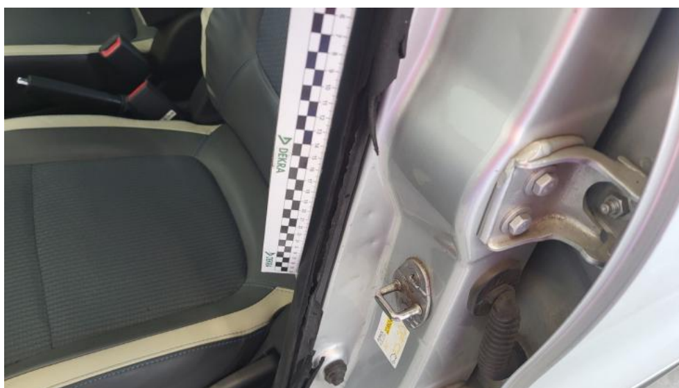
Fot. 72. Uszczelka drzwi przednich L - Pęknięcie/rozerwanie 1
