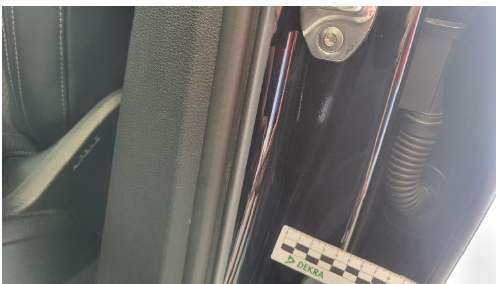
Fot. 82. Słupek środkowy L - Wgniecenie/odkształcenie 1
