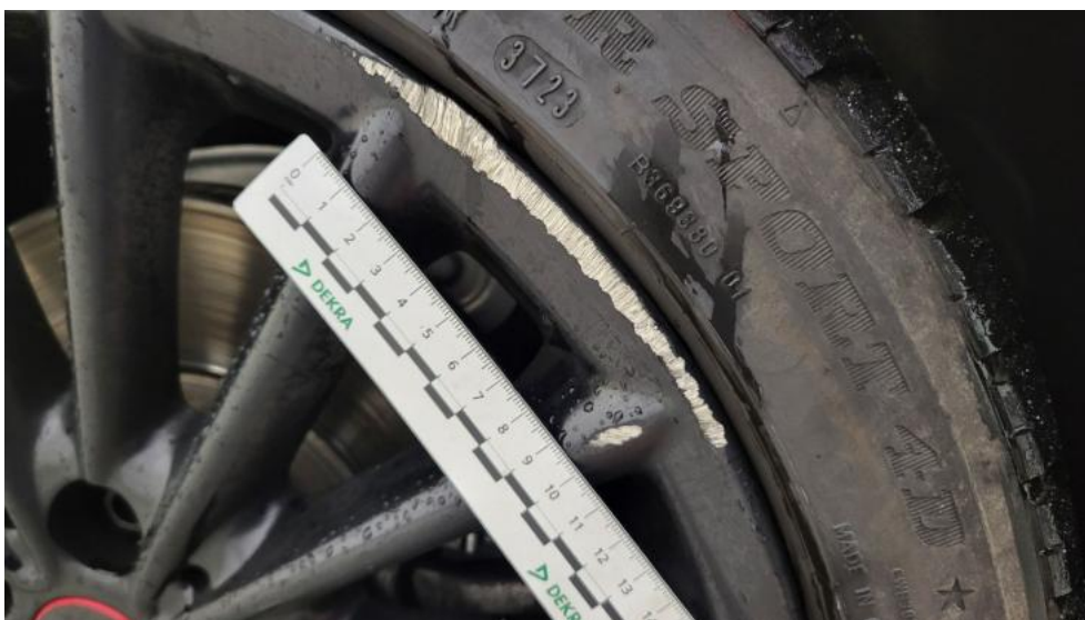
Fot. 42. Felga aluminiowa przednia P - Rysa/odprysk 1
