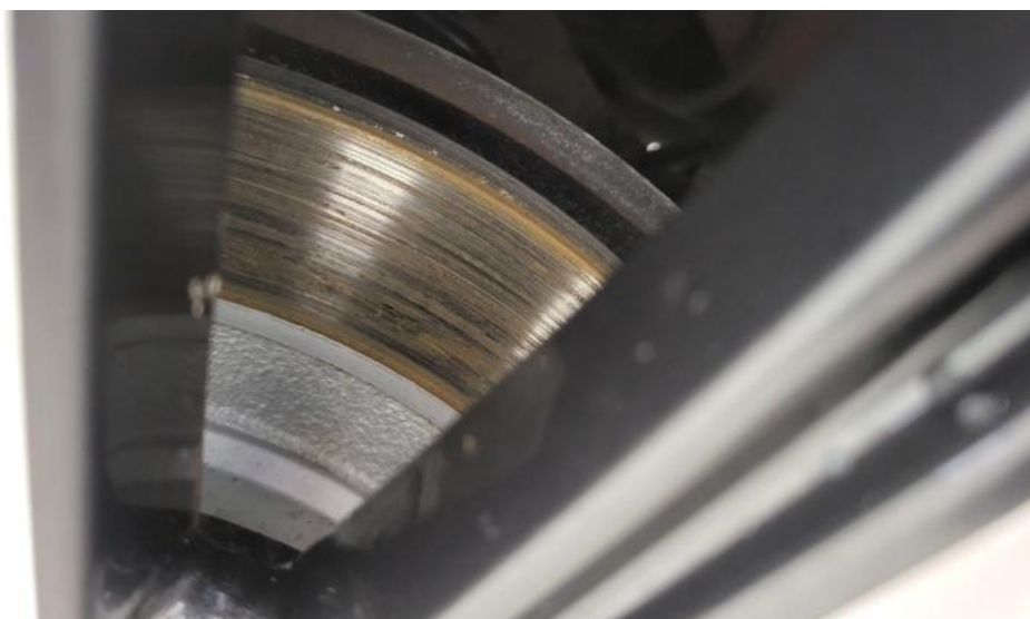
Fot. 16. Tarcza hamulcowa tylna prawa
