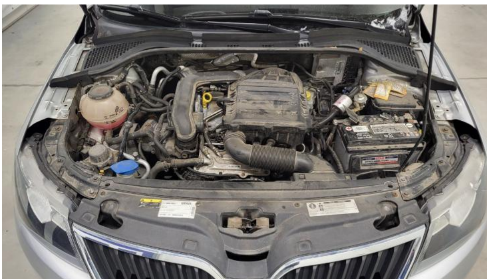
Photo 17. Komora silnika
